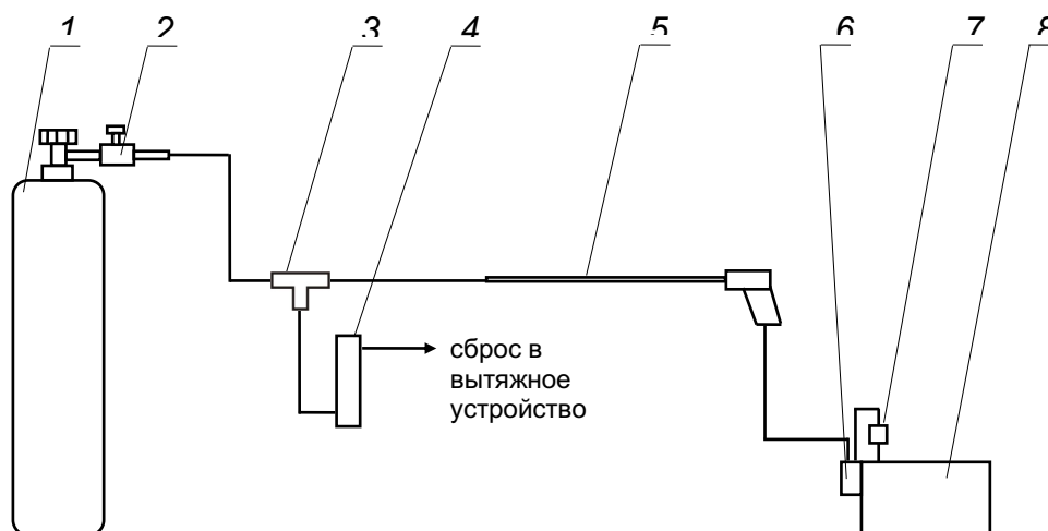
Рисунок 10 – Газовая схема соединений при калибровке нулевых показаний газоанализатора по нулевой газовой смеси из баллона под давлением и контроле точности результатов измерений по ПГС
